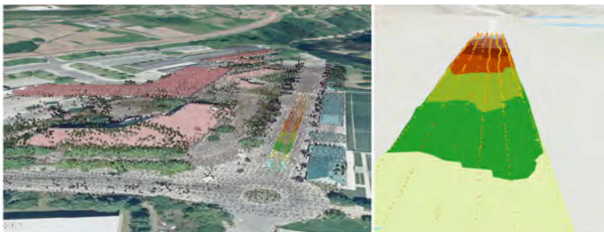
Nube de puntos GPR (espesor de firme) e MDE sobre nube de puntos LiDAR
